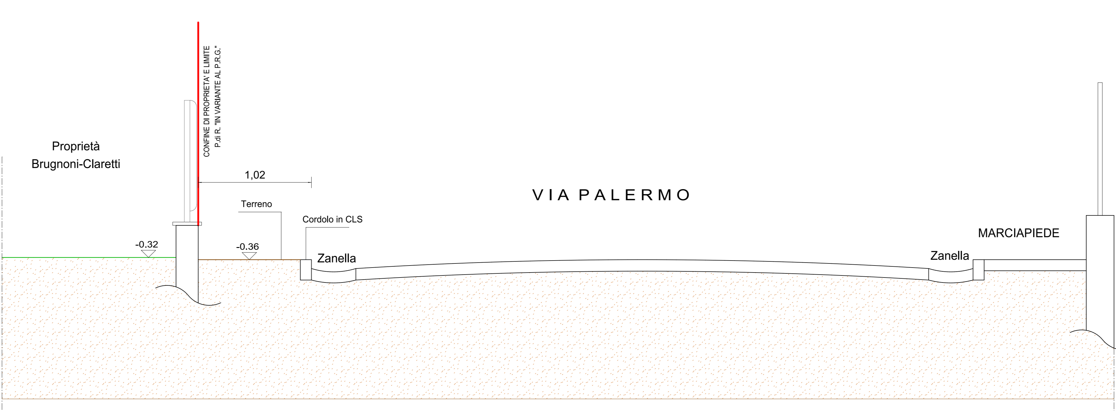
SEZIONE B-B STATO ATTUALE SCALA 1:20
