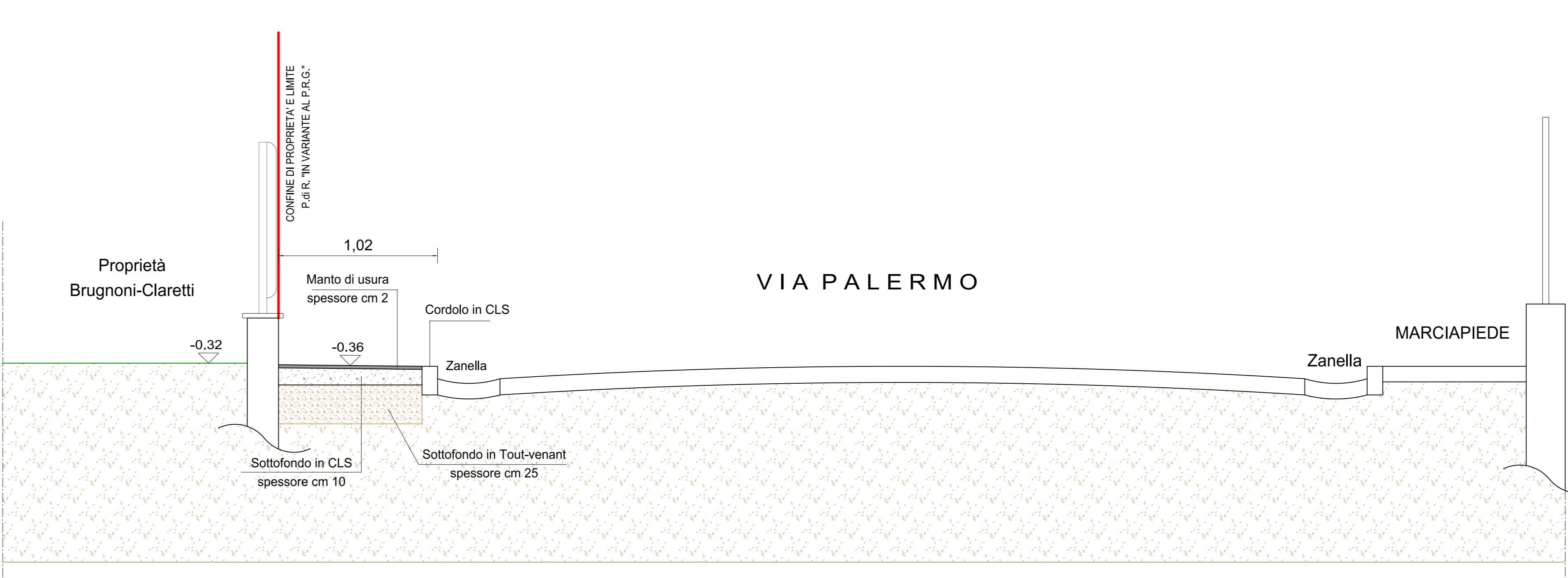
SEZIONE B-B STATO DI PROGETTO SCALA 1:20
