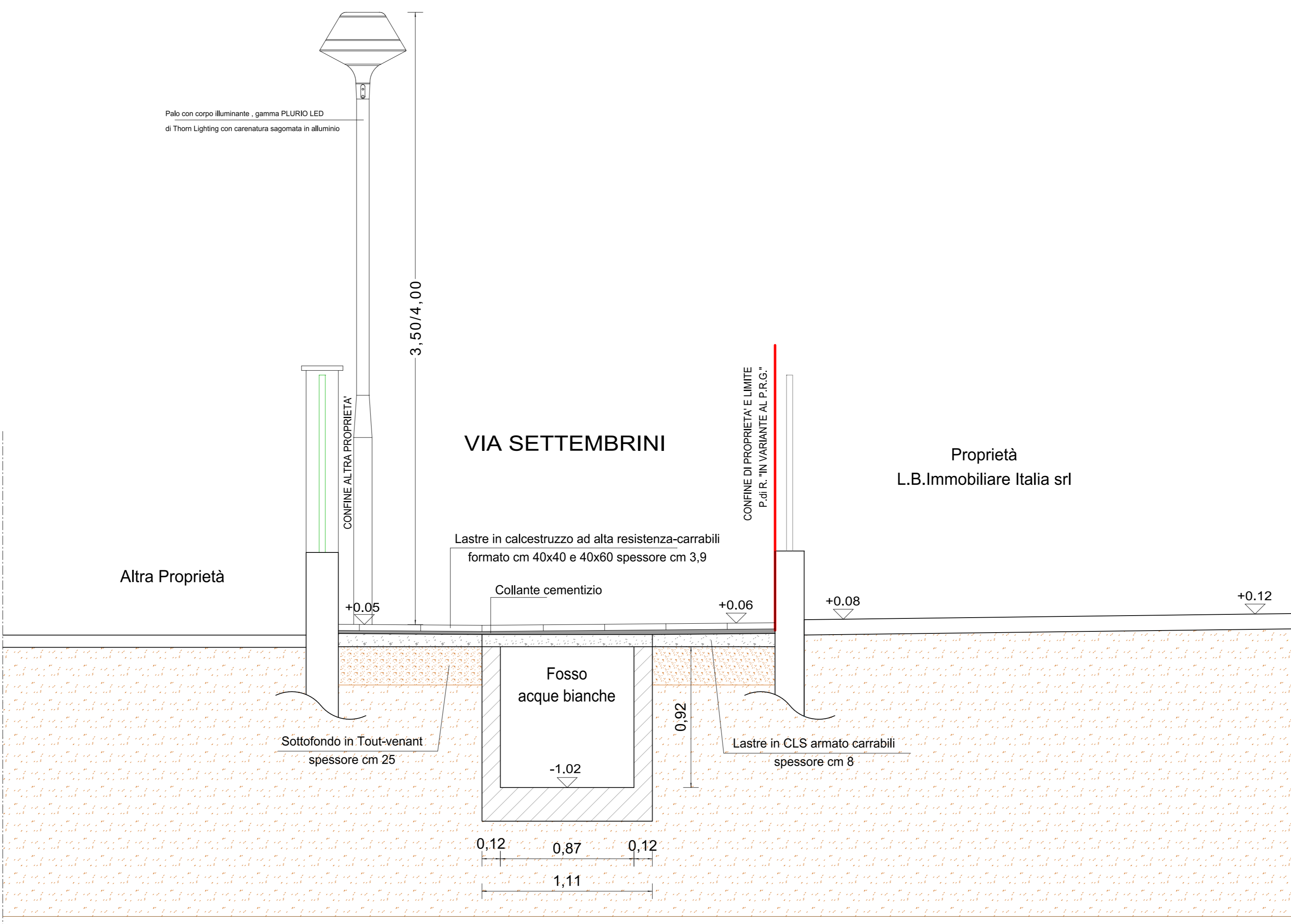
SEZIONE A-A STATO DI PROGETTO SCALA 1:20
