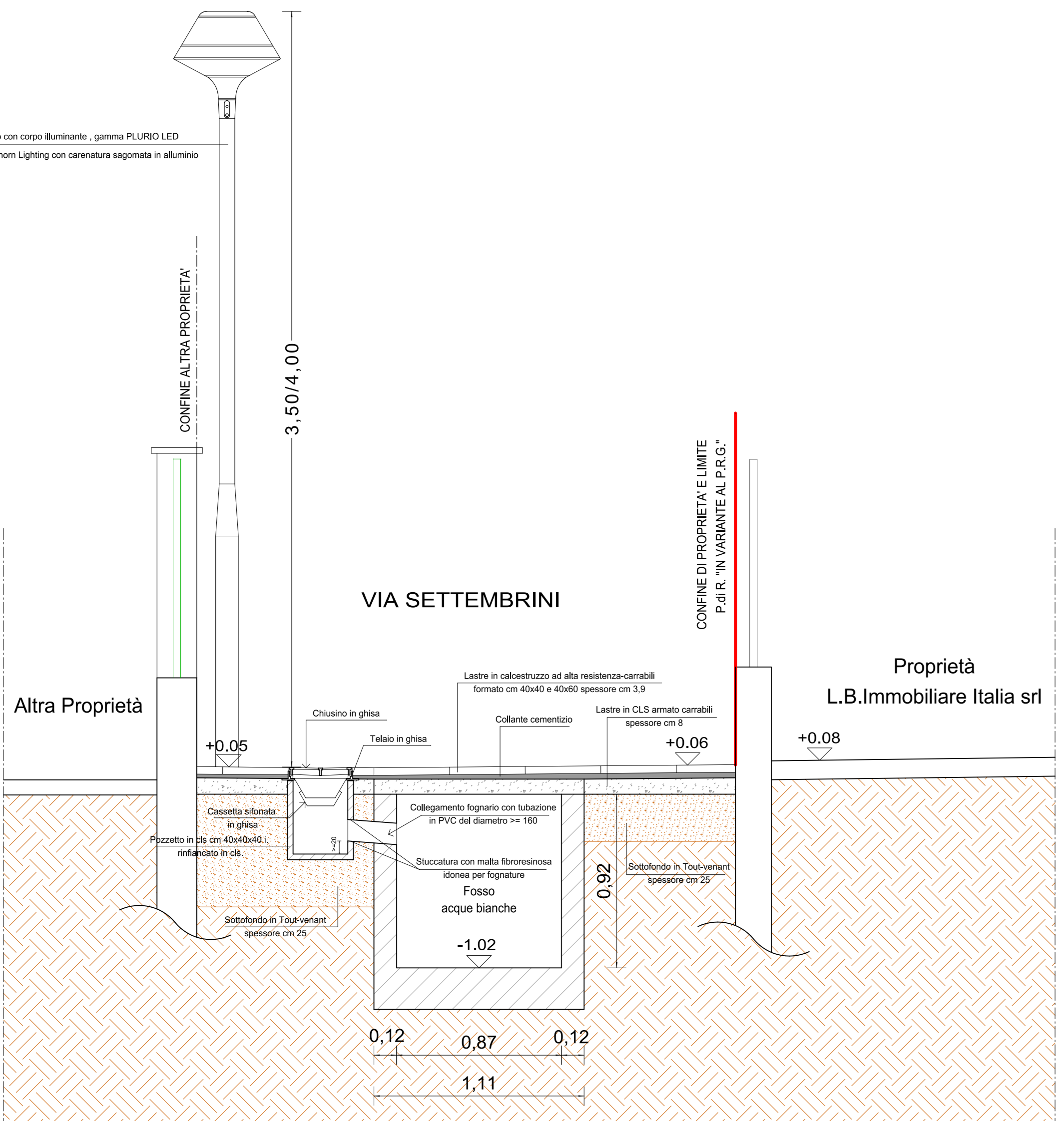
PARTICOLARE CADITOIA STRADALE A SIFONE E PALI ILLUMINAZIONE STATO DI PROGETTO SCALA 1:20
