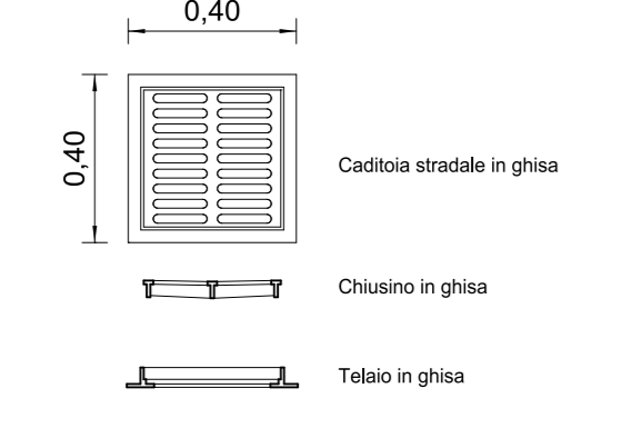
PARTICOLARE CADITOIA STRADALE A SIFONE E PALI ILLUMINAZIONE STATO DI PROGETTO SCALA 1:20
