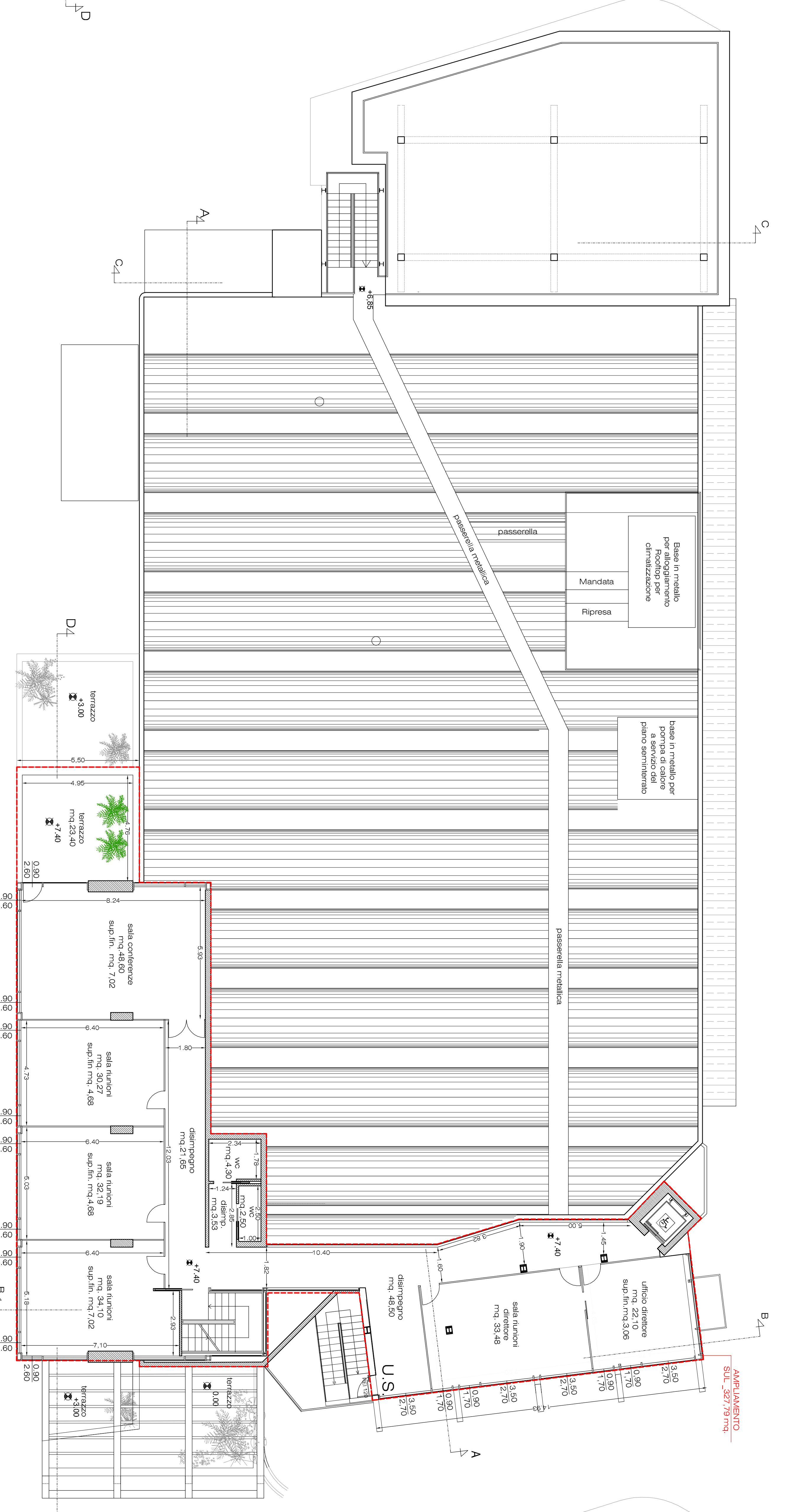
PLANIMETRIA PIANO SECONDO
