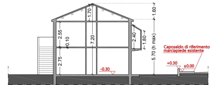
Sezione C-C
