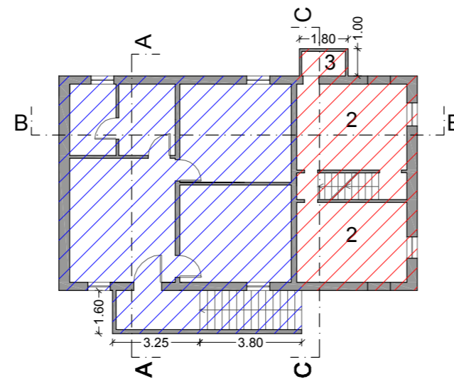
Piano Primo
