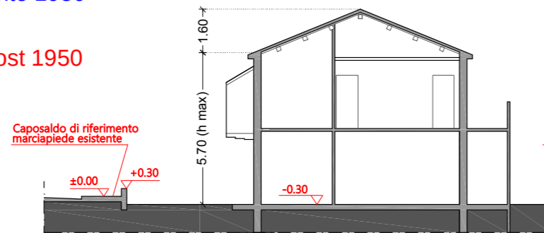
Sezione A-A
