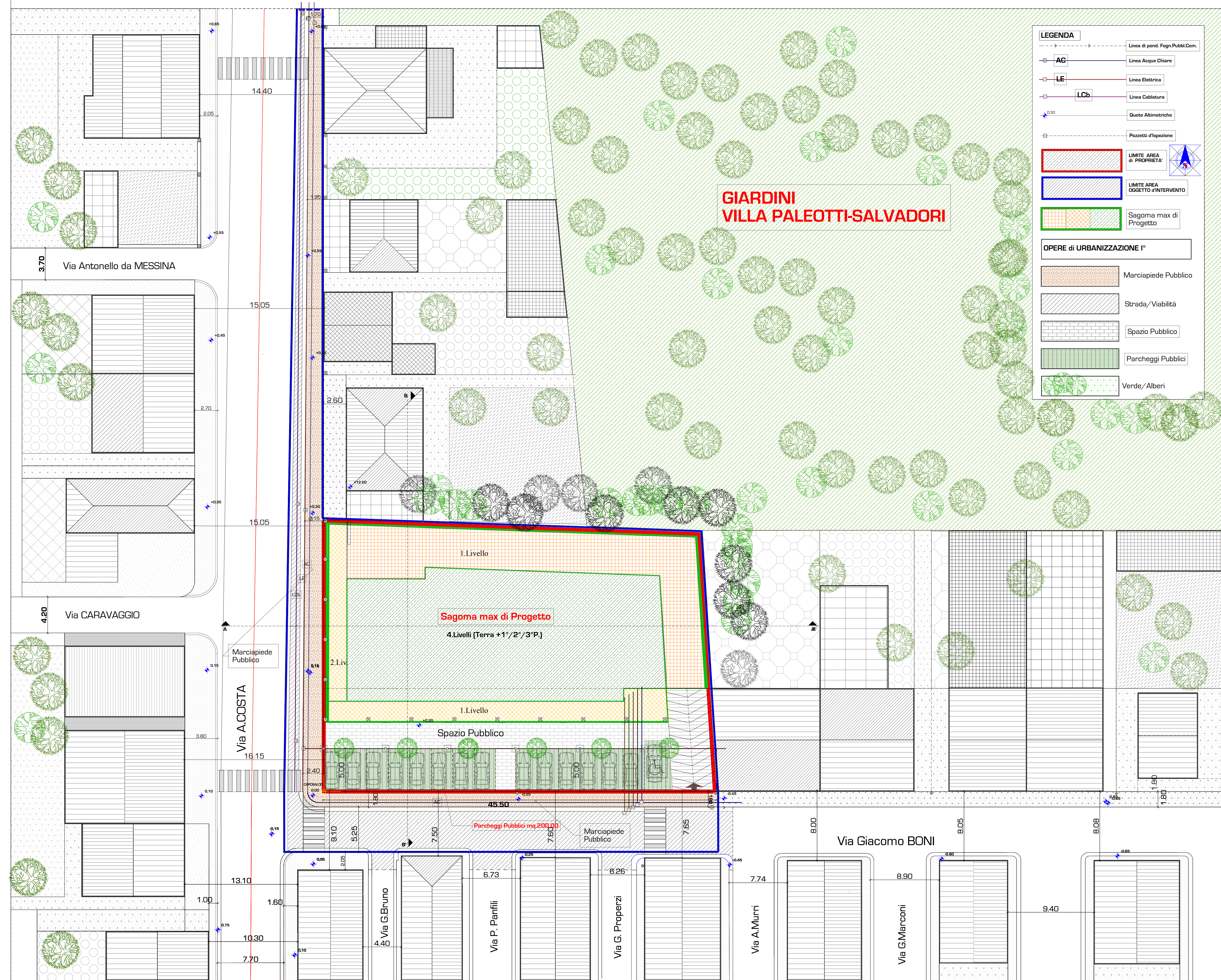
PLANIMETRIA GENERALE - Area d'INTERVENTO - OPERE di URBANIZZAZIONE I° 1/200
