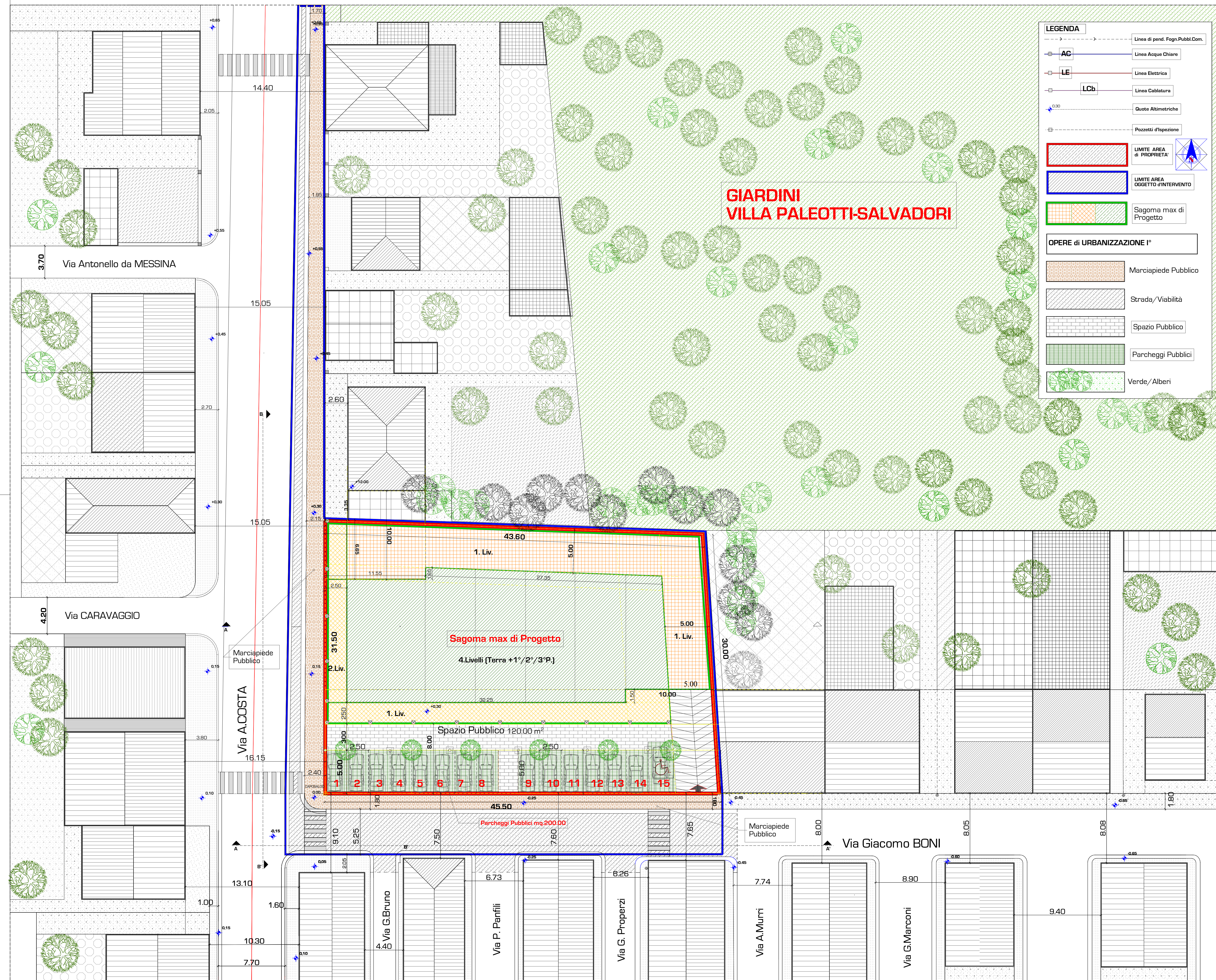
PLANIMETRIA GENERALE - PROFILI E QUOTE. 1/200
