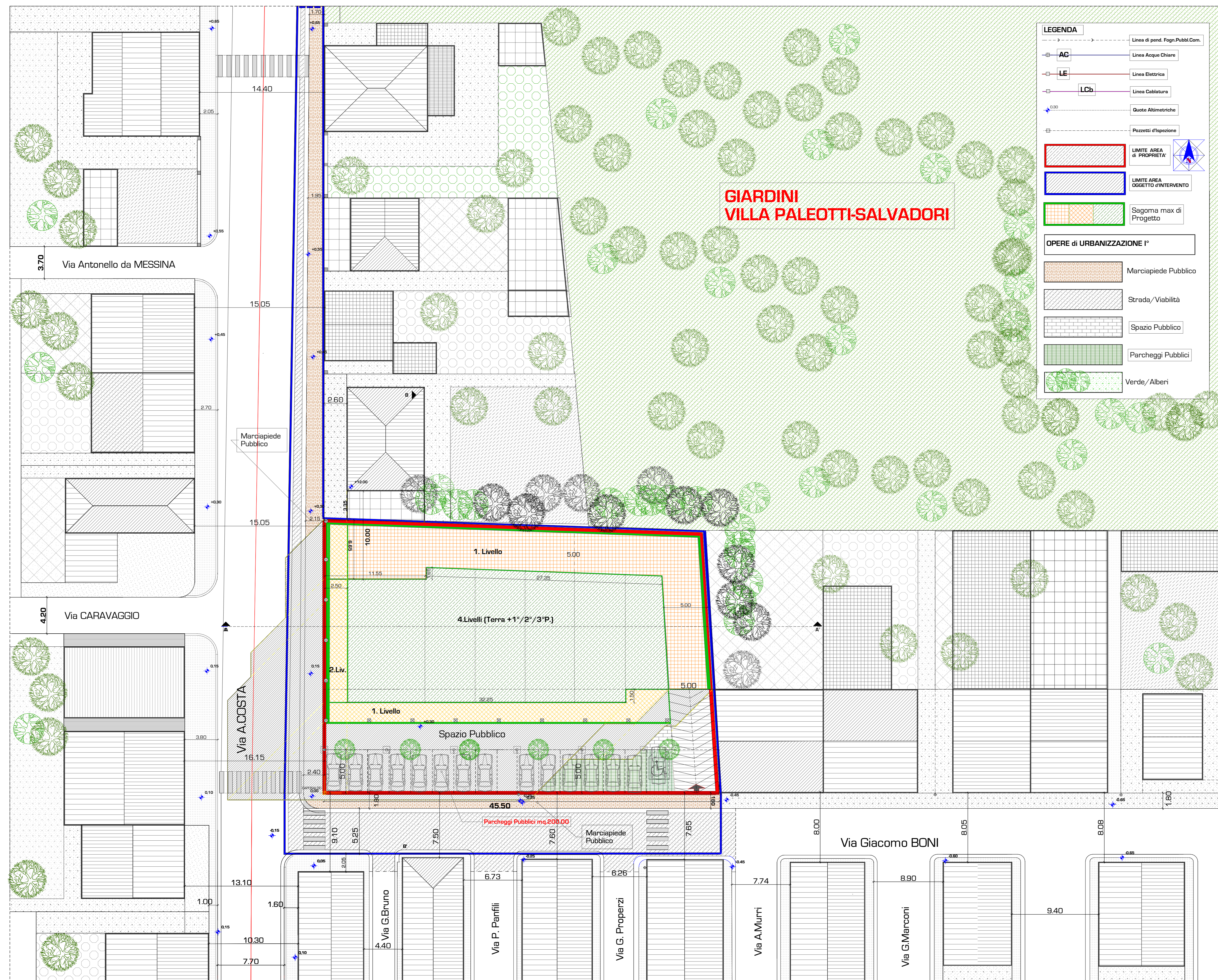
PLANIVOLUMETRICO/SEZIONI - AREA di PROGETTO 1/200
