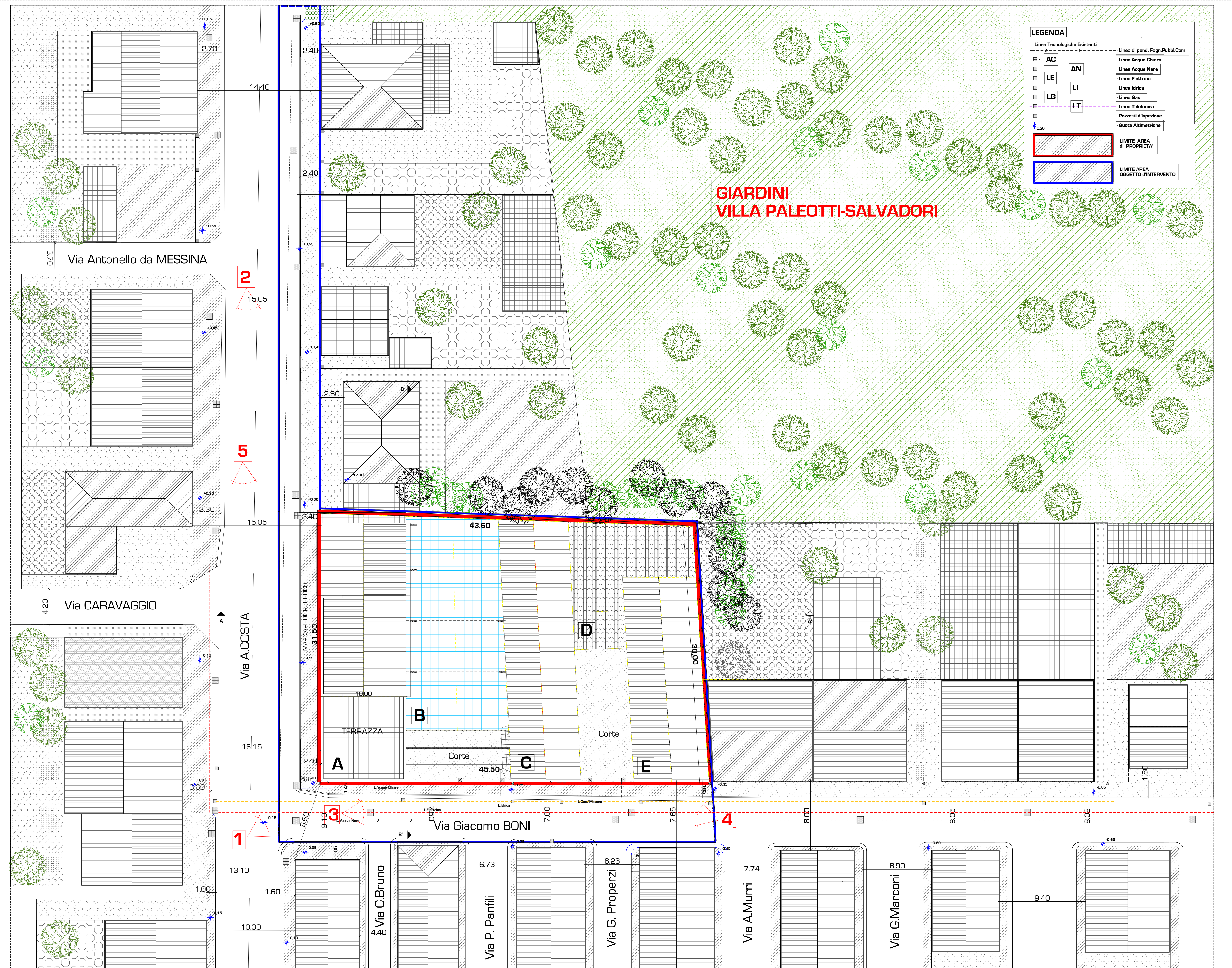
PLANIMETRIA GENERALE - PUNTI di VISTA Fotografici - STATO ATTUALE -1/200
